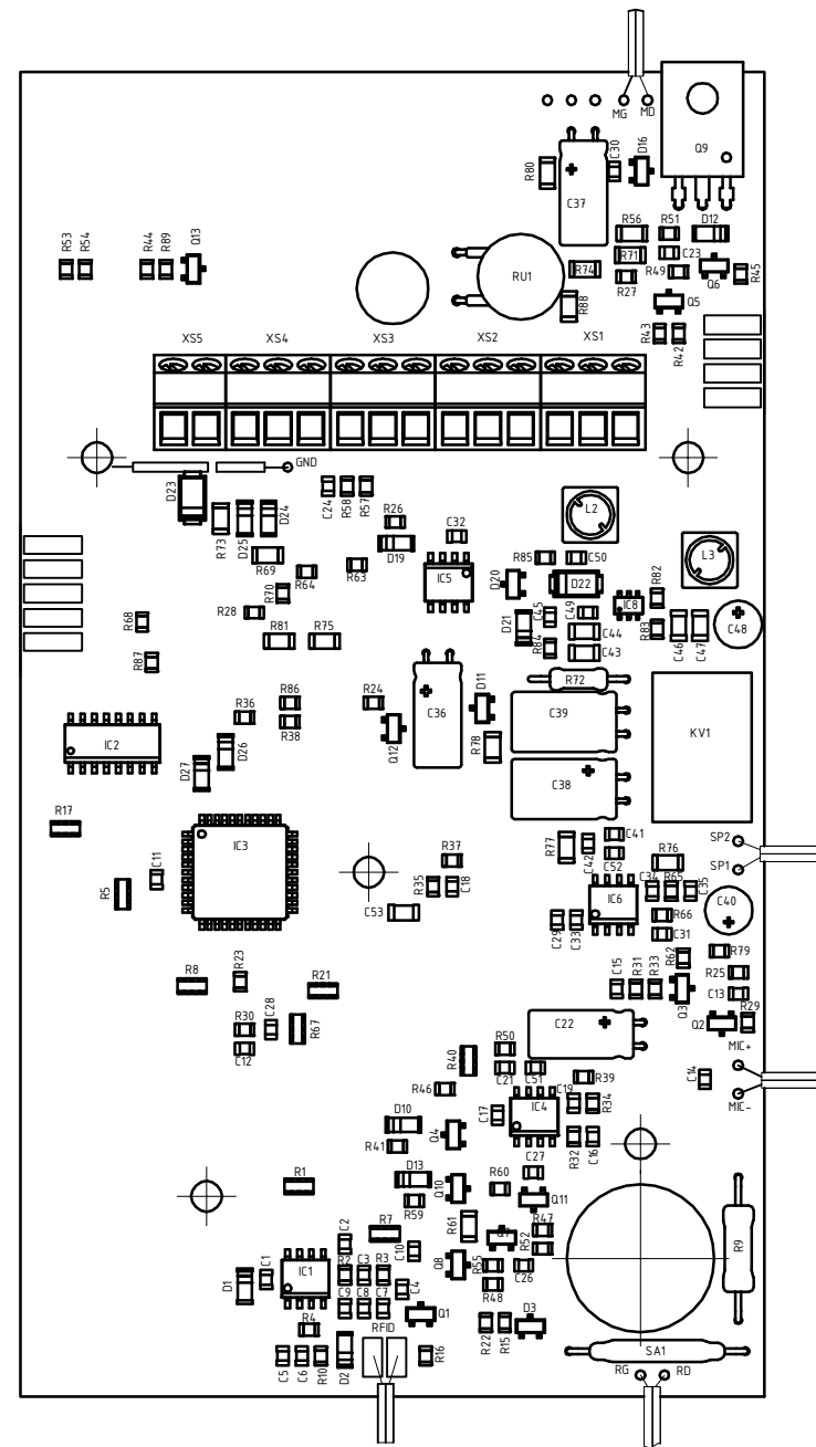
Плата БВД-М202RTCP Сборочный чертеж
