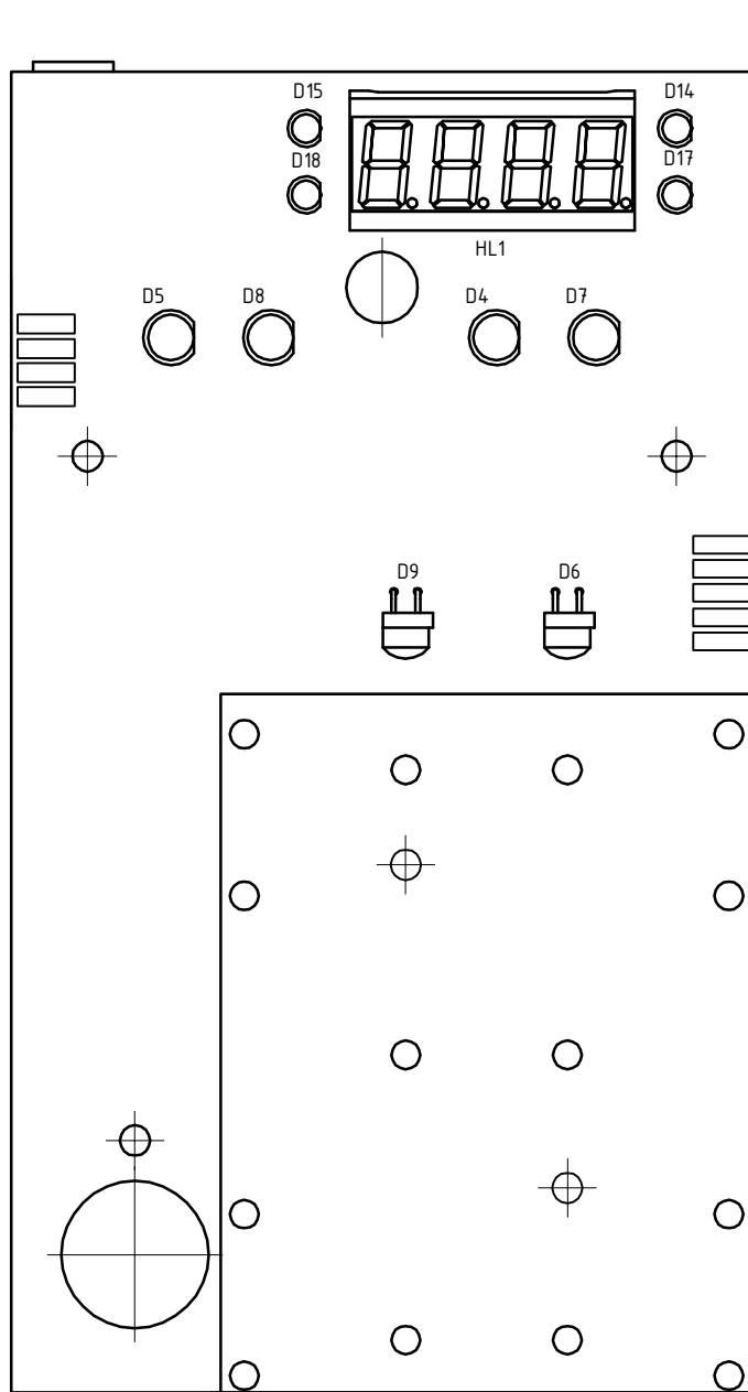
Плата БВД-М202RTCP Сборочный чертеж
