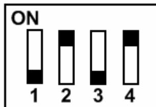
Рис.12 Положение движков переключателя конфигурации при работе с БВ «VIZIT» без коммутатора типа КМВ1.4-2.4(М).
