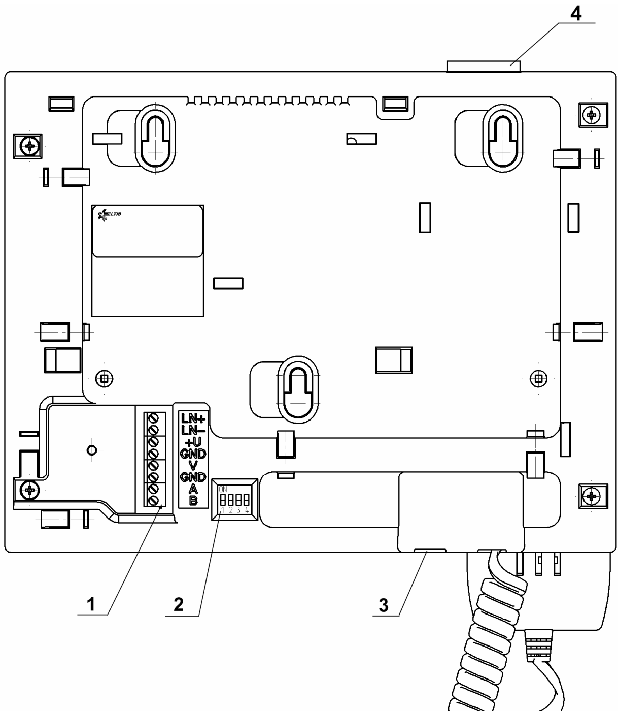
Рис.2: Вид с обратной стороны видеомонитора.
