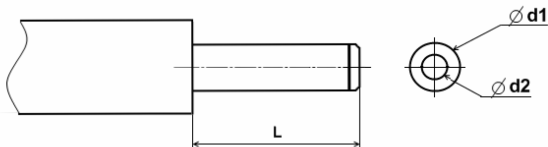
Рис.4 Штекер для дополнительного разъема питания видеомонитора: d1=5,0\dots6,0 мм; d2=2,0\dots2,5 мм; L=9\dots13 мм.
