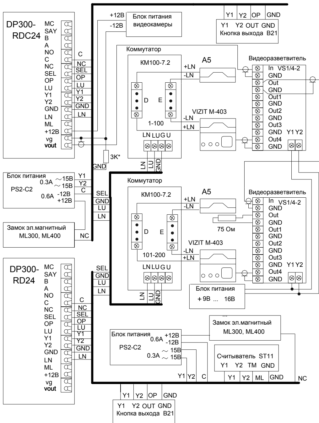
Рис.3 Пример схемы подключения DP300-RDC24 в составе домофонного комплекса.
