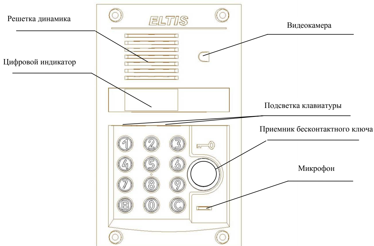
Рис.1 Внешний вид со стороны лицевой панели блока вызова DP300-RDC24.
